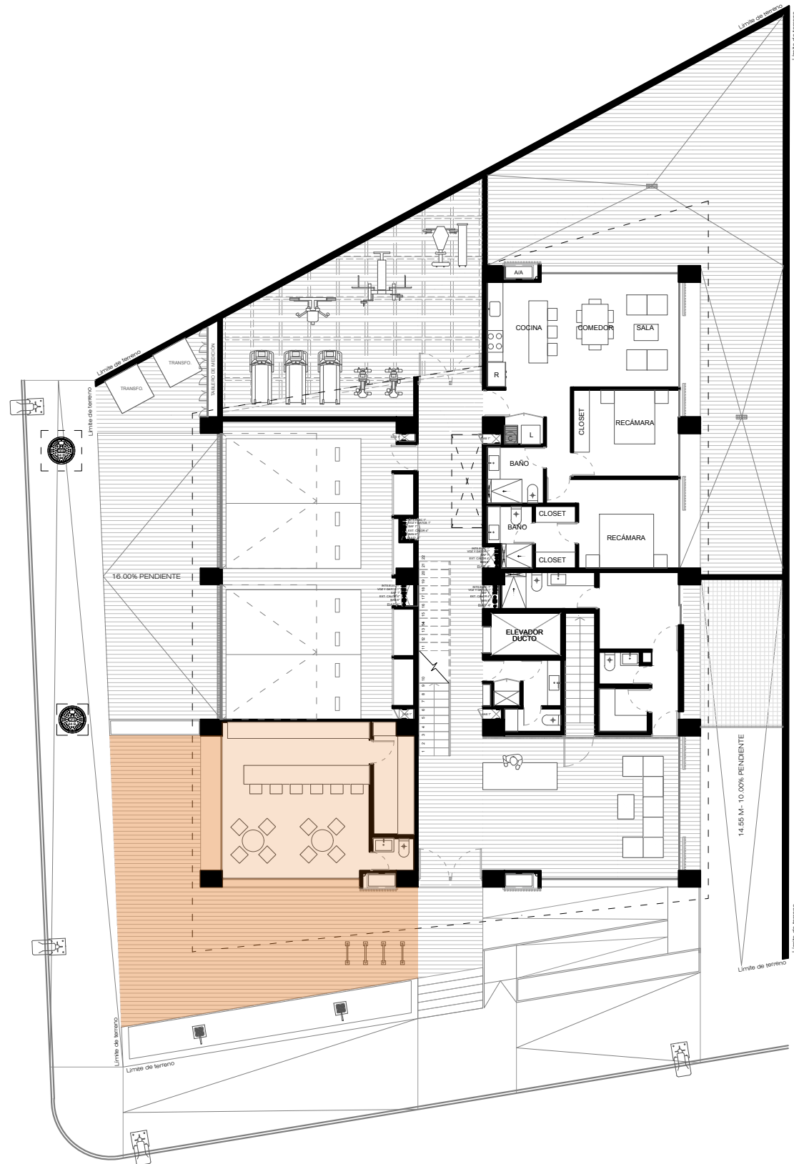
PLANTA BAJA GENERAL - 1/200
